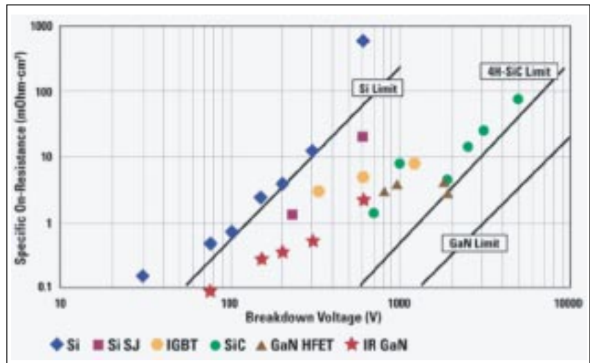
圖 1：IR GaN 技術大幅提升功率元件的 FOM 值，圖為 Si、SiC、IGBT 與 GaN HFET 與 IR GaN 技術在導通電阻值的比較結果。
